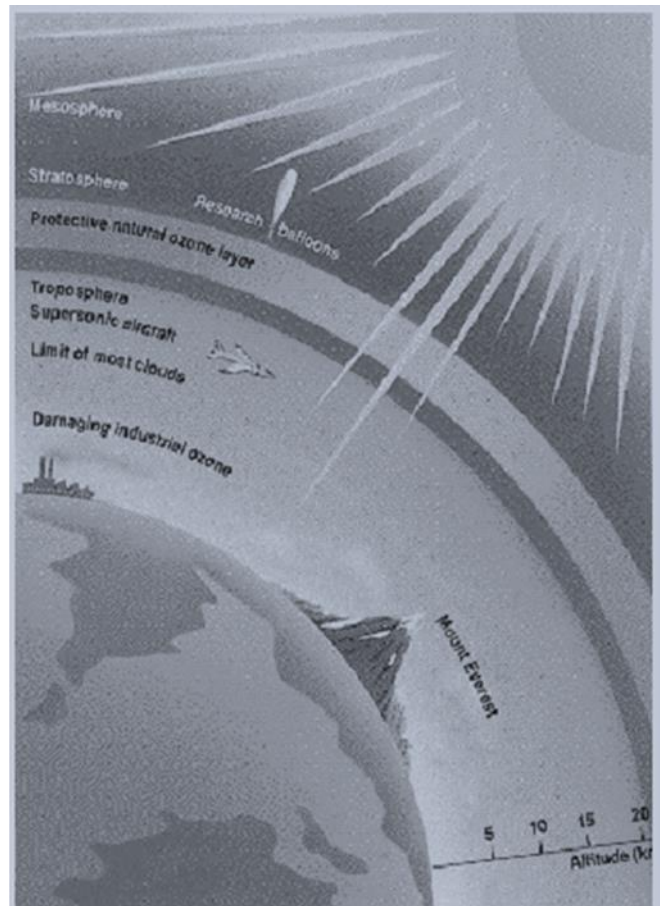
Fig: 2.1: the ozone layer
